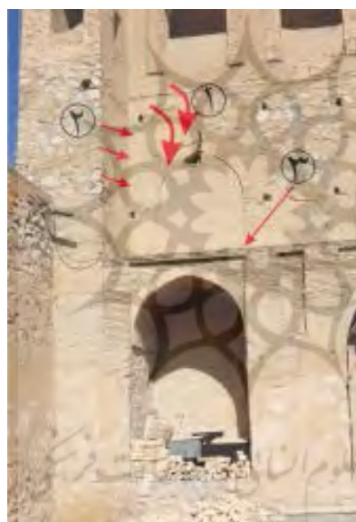
تصویر ۱۳: نمایش شماتیک کنش چرخش دیوار و واکنش برج و کمربند الحاقی. ۱- محل چرخش دیوار، ۲- نیروی وارده برج به بخش آسیب دیده، ۳- کمربند الحاقی برای جلوگیری از چرخش بیشتر بنا (نگارندگان، ۱۳۹۵).
