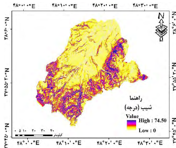
شکل ۲: نقشه شیب حوضه آبخیز کوزه‌تپراقی
