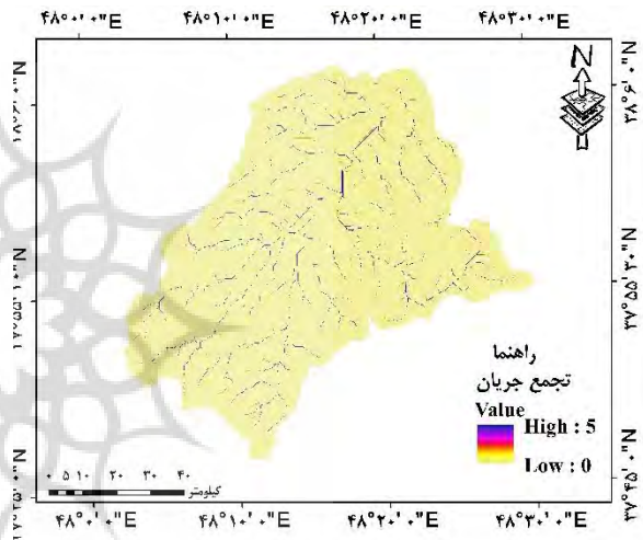
شکل ۴: نقشه تجمع جریان حوضه آبخیز کوزه‌تپراقی
