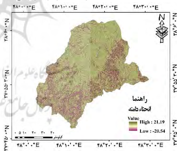
شکل ۸: نقشه انحناء دامنه حوضه آبخیز کوزه‌توپراقی
