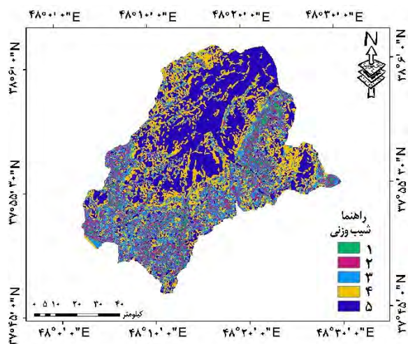
شکل ۳: نقشه شیب وزنی حوضه آبخیز کوزه‌تپراقی
