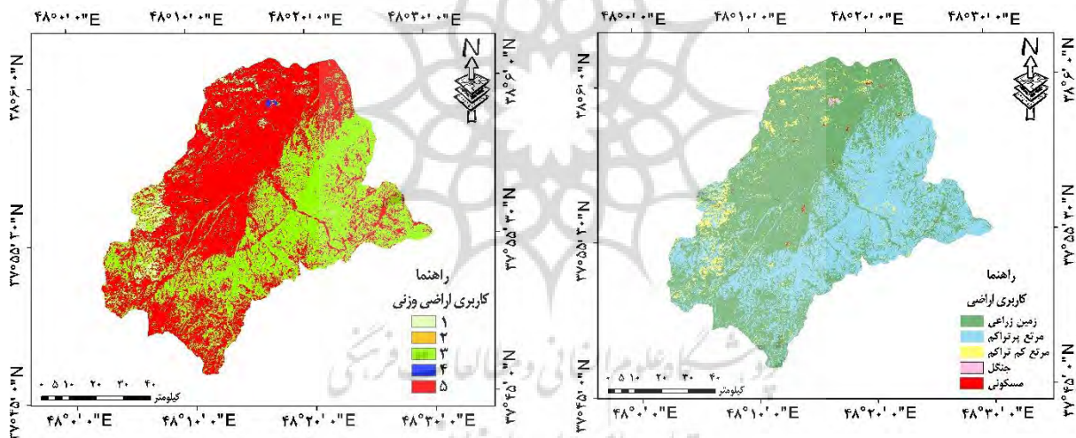
شکل ۱۰: نقشه کاربری اراضی حوضه آبخیز کوزه توپراقی
