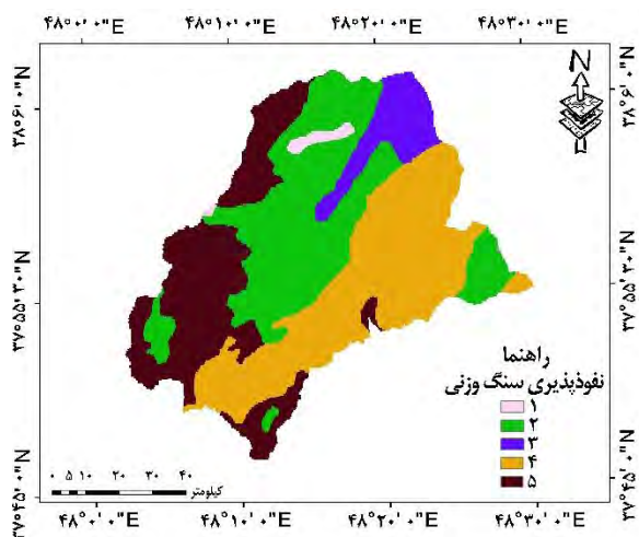
شکل ۱۳: نقشه نفوذپذیری سنگ وزنی حوضه آبخیز کوزه توپراقی
