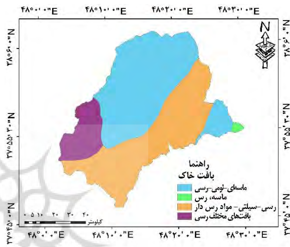
شکل ۶: نقشه بافت خاک حوضه آبخیز کوزه‌توپراقی
