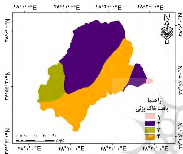
شکل ۷: نقشه بافت خاک وزنی حوضه آبخیز کوزه‌توپراقی
