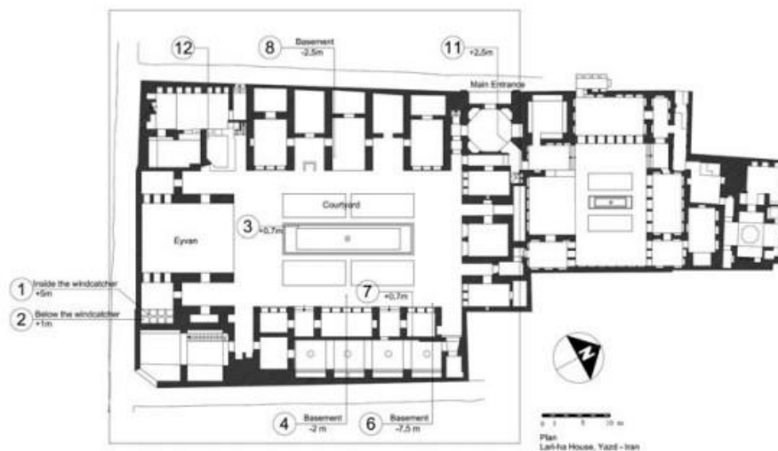
شکل ۸ پلان خانه لاری‌ها و محل قرارگیری دیتالاگرها
