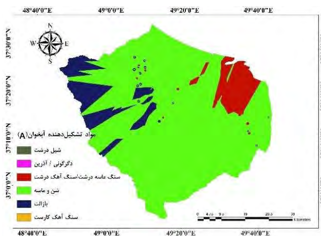
شکل ۶. لایه محیط آبخوان
