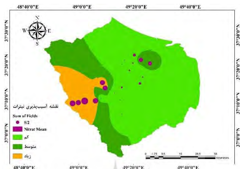
شکل ۱۳. نقشه آسیب‌پذیری منطقه بر اساس غلظت نیترات ۲۰ چاه
