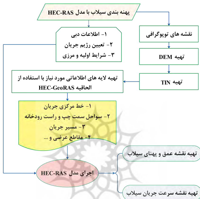
شکل ۳: فلوچارت پهنه‌بندی سیلاب بر اساس مدل HEC-RAS
