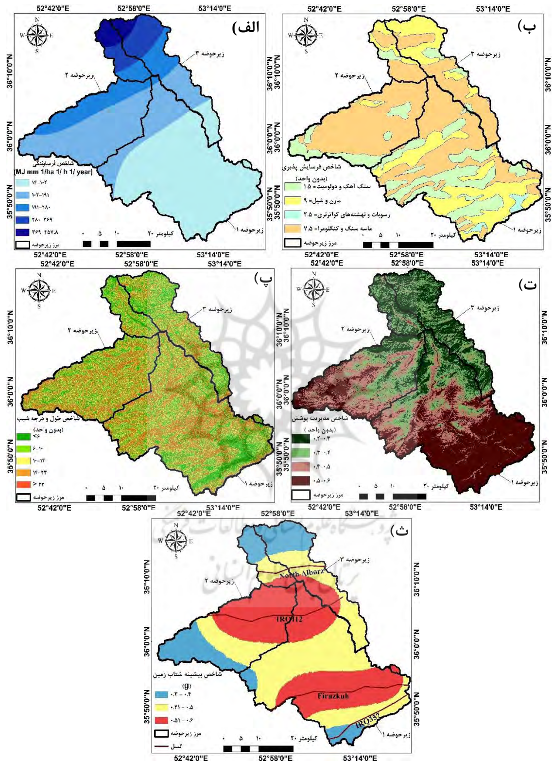
شکل ۳: شاخص‌های فرسایش در معادله RUSLE (الف) فرساینده‌گی (ب) فرسایش پذیری (پ) طول و درجه شیب، (ت) مدیریت پوشش (ث) بیشینه شتاب زمین
