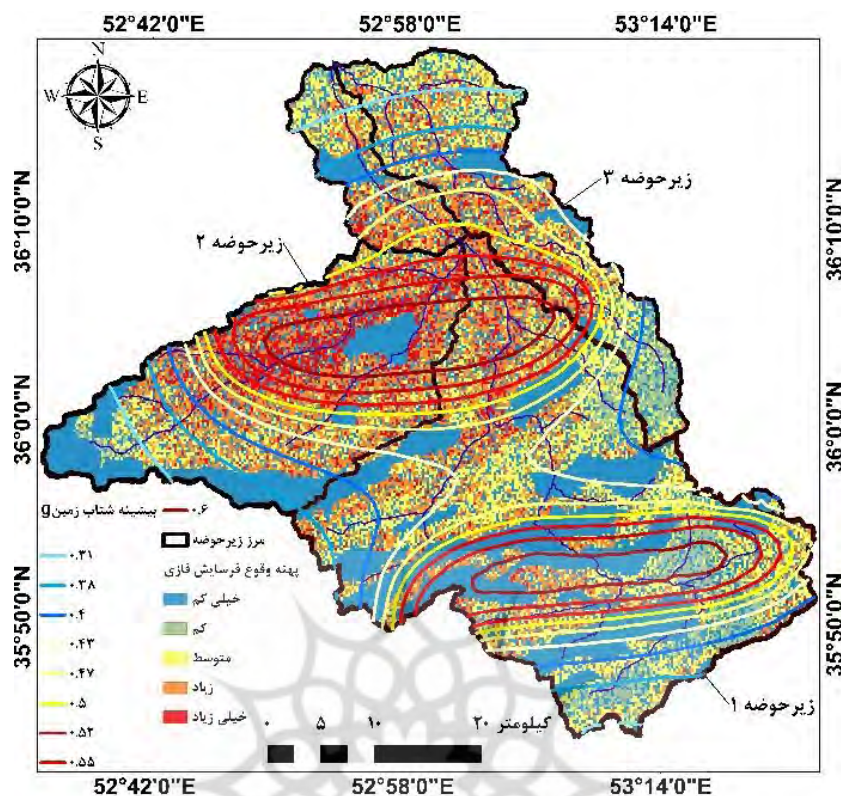
شکل ۵: نقشه پهنه‌بندی وقوع فرسایش به روش منطق فازی
