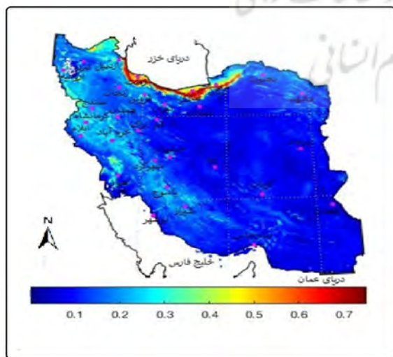
نگاره ۲: توزیع مکانی میانگین NDVI
