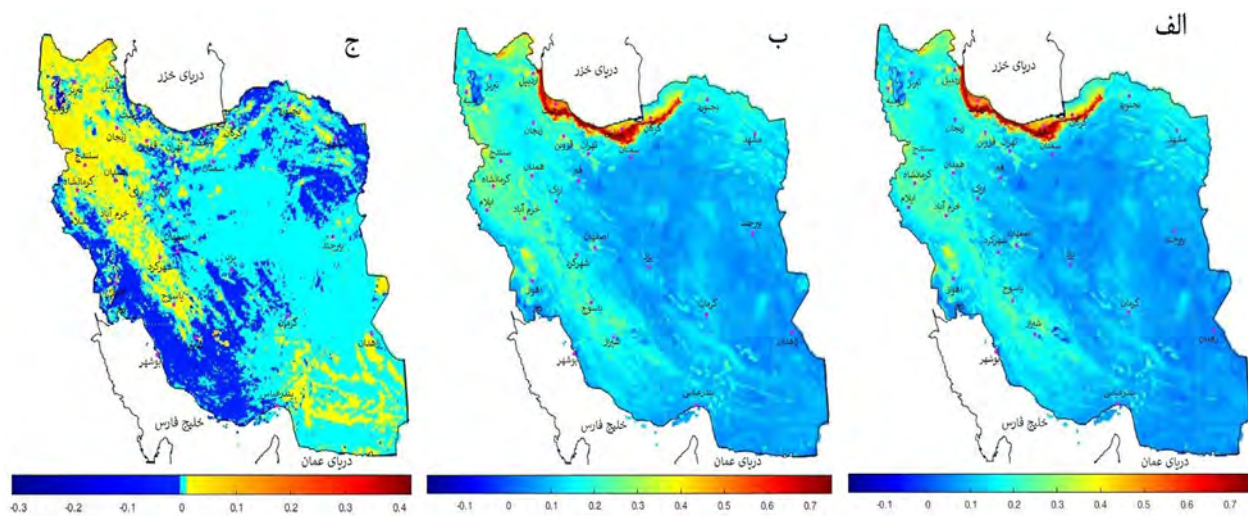
نگاره ۳: مقادیر نمایه NDVI برای: الف) نیم دوره اول (۲۰۰۸-۲۰۱۱)، ب) نیم دوره دوم (۲۰۱۶-۲۰۰۹)، ج) تفاضل آن‌ها
