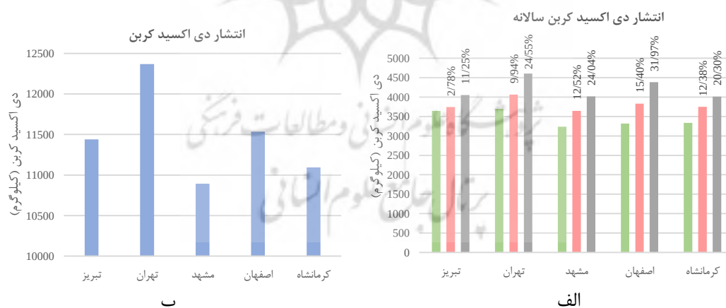
نمودار ۴. مقایسه میزان گاز دی‌اکسیدکربن منتشرشده در پنج شهر: الف) انتشار دی‌اکسیدکربن سالانه در سال‌های ۲۰۳۰، ۲۰۶۰ و ۲۰۹۰، ب) مجموع گاز دی‌اکسیدکربن منتشرشده در سال‌های ۲۰۳۰، ۲۰۶۰ و ۲۰۹۰.
