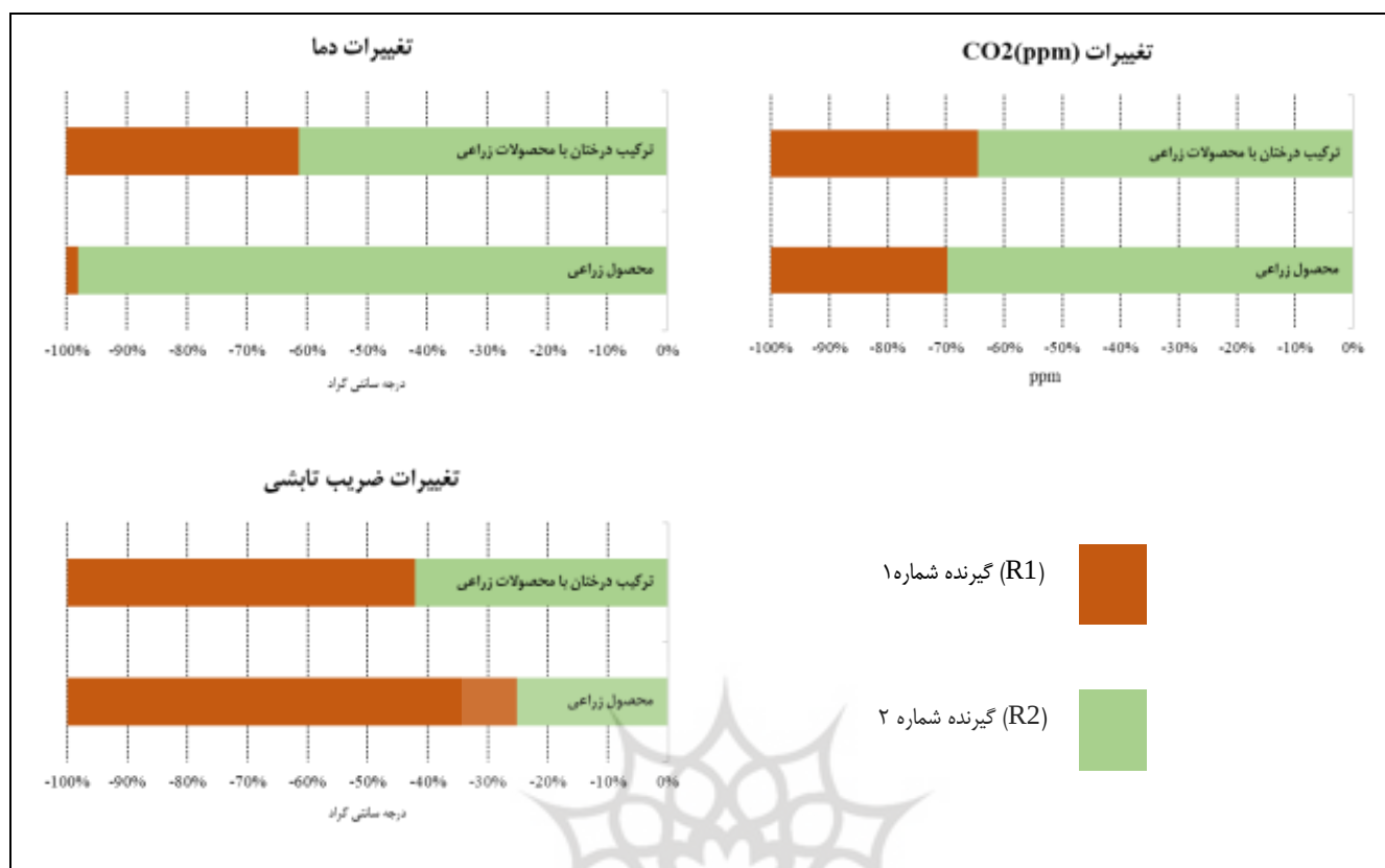
شکل ۹: تغییرات مقدار دما، ضریب تابشی و CO 2 در سناریوها، در مدت ۸ ساعت شبیه سازی در ارتفاع ۱/۸ متری (درگیرنده شماره ۲)
