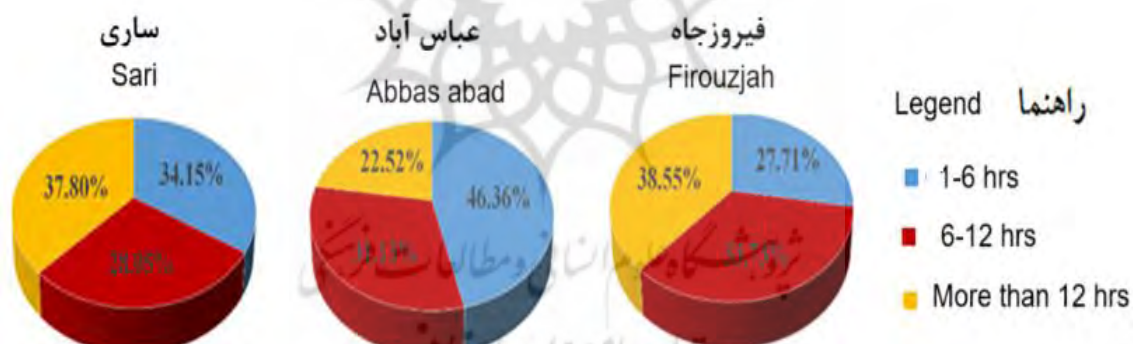
شکل ۳- درصد رگبارهای مورد مطالعه در هر یک از کلاس‌های بارشی برای ایستگاه‌های باران‌سنجی منتخب Fig. 3. Percentage of studied storms in each of the rainfall classes in the selected rain gauge stations
