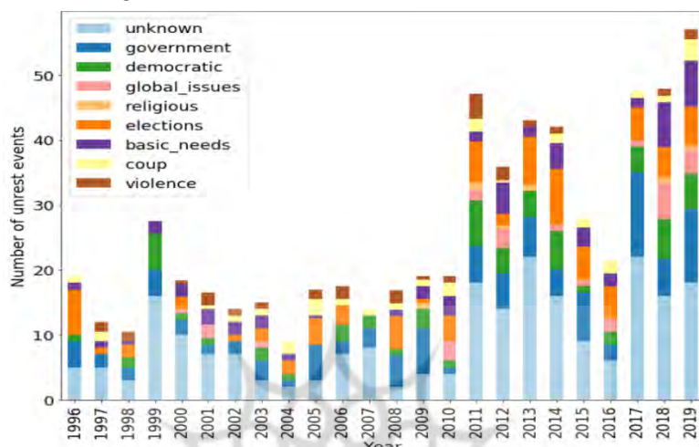
شکل ۳: رویدادهای ناآرامی اجتماعی از سال ۱۹۹۶ الی ۲۰۱۹ ۱
