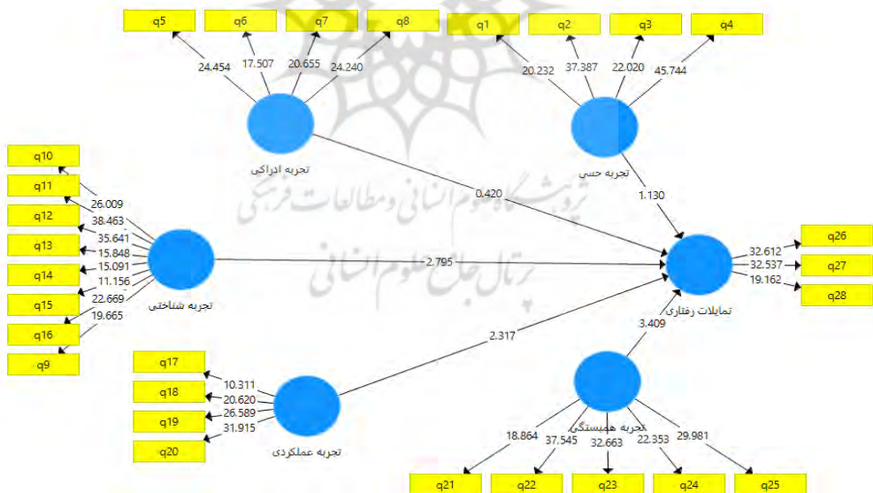
شکل ۱. نتایج بارهای عاملی بین سؤالات و متغیرها و همچنین ضرایب مسیر بین متغیرها
