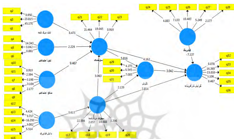
شکل ۲. مدل تحقیق در حالت معناداری ضرایب (t-value)
