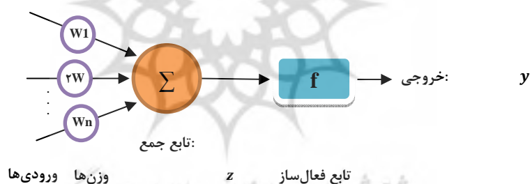
شکل ۱. ساختار نورون مصنوعی
