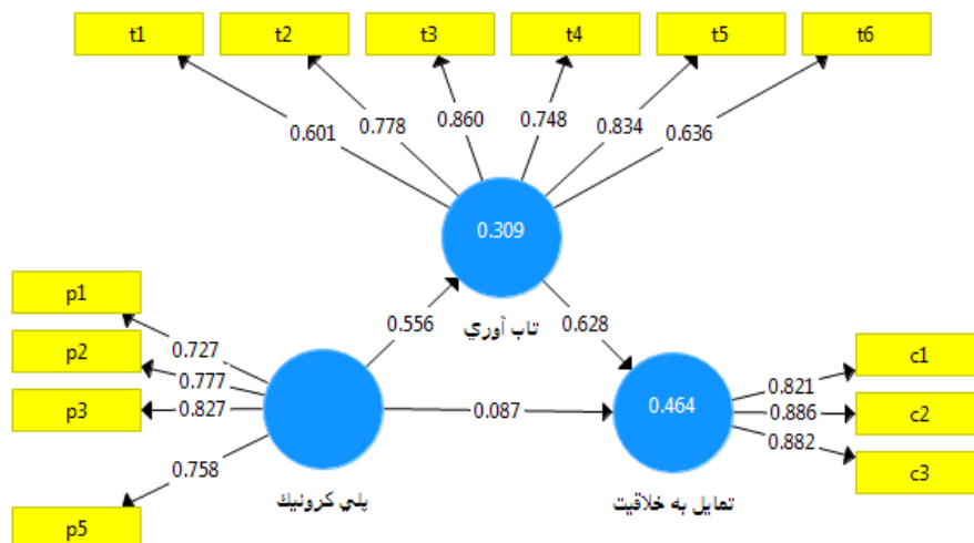
شکل ۳. مقدار R^2
