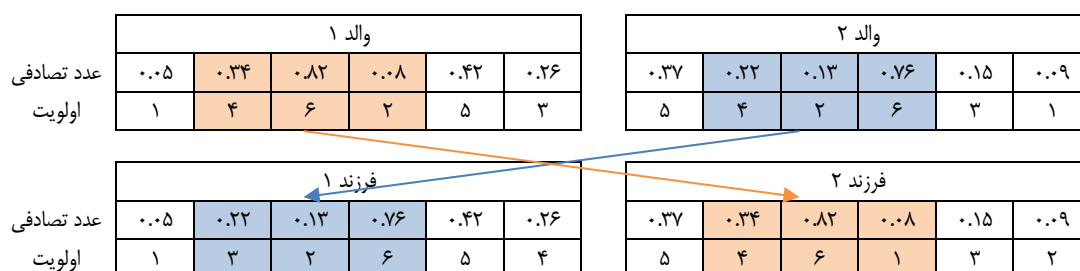
شکل ۷. مکانیسم عملگر ترکیب دو نقطه‌ای
