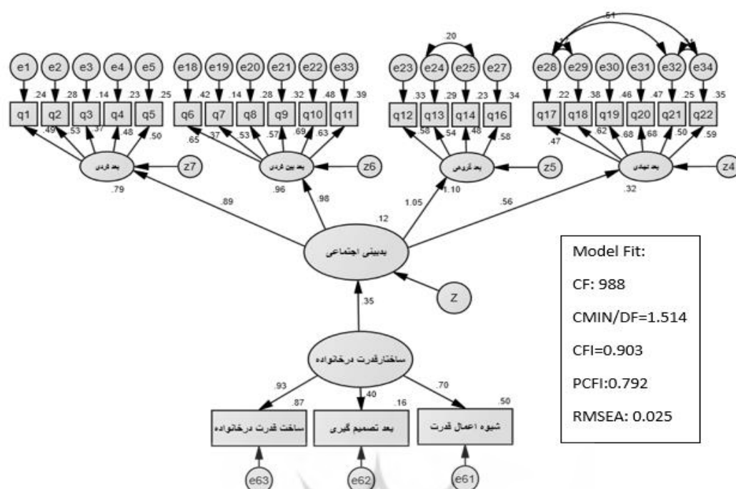
شکل ۲- مدل ساختاری
