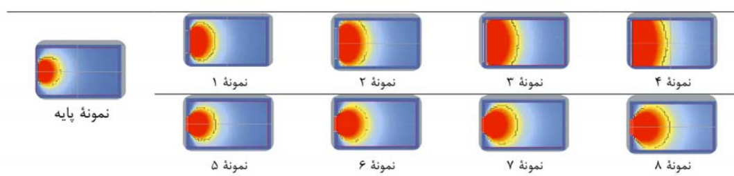
تصویر ۶. کانتور نور روز در نمونه‌های موردی با کشیدگی متفاوت بازشو. مأخذ: نگارندگان.
