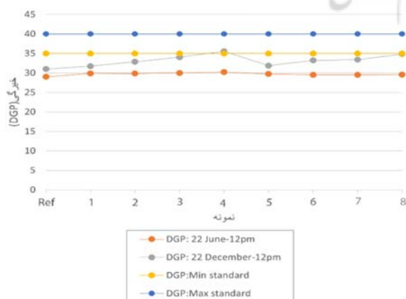
تصویر ۸. نتایج عددی شاخص خیرگی در نمونه‌های موردی با کشیدگی متفاوت بازشو. مأخذ: نگارندگان.
