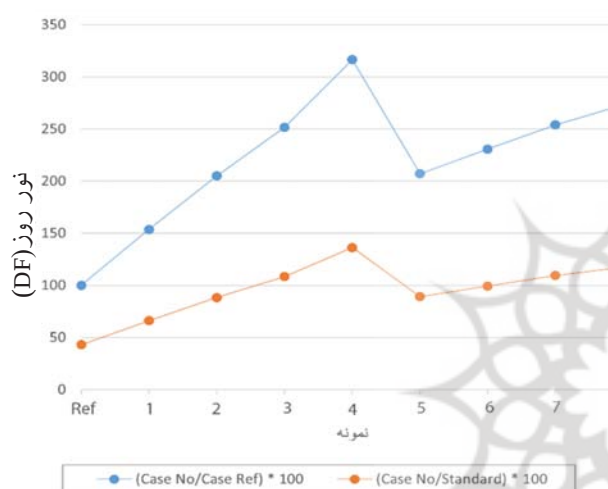
تصویر ۴. نتایج عددی شاخص نور روز در نمونه‌های موردی با کشیدگی متفاوت بازشو. مأخذ: نگارندگان.
