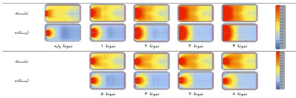
تصویر ۱۲. نتایج عددی شاخص دید به بیرون در نمونه‌های موردی با کشیدگی متفاوت بازشو. مأخذ: نگارندگان.
