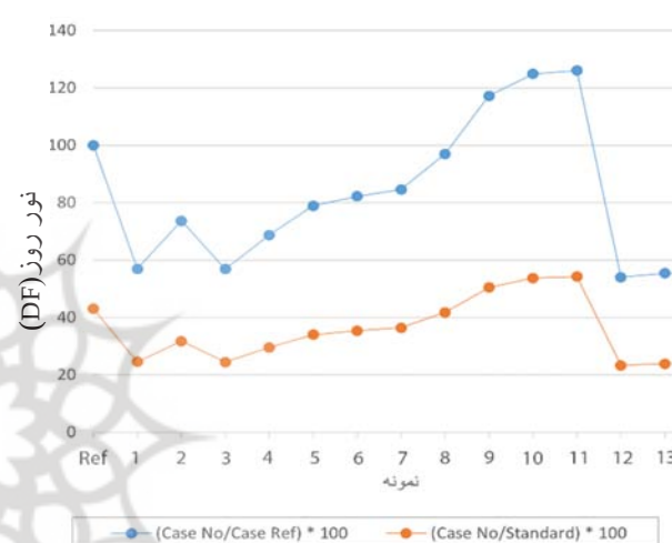
تصویر ۳. نتایج عددی شاخص نور روز در نمونه‌های موردی با موقعیت متفاوت بازشو. مأخذ: نگارندگان.
