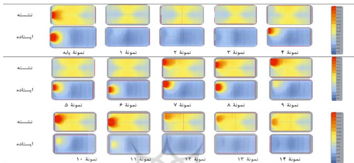
تصویر ۹. کانتور دید به محیط بیرون در نمونه‌های موردی با موقعیت‌های متفاوت بازشو. مأخذ: نگارندگان.
