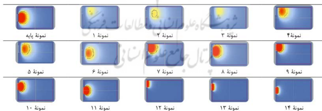
تصویر ۵. کانتور نور روز در نمونه‌های موردی با موقعیت‌های متفاوت بازشو. مأخذ: نگارندگان.
