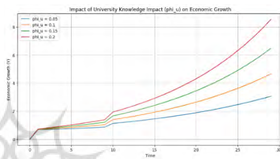
شکل ۴. شبیه‌سازی برای حالات مختلف \phi_u و شبیه‌سازی مونت کارلو با فاصله اعتماد ۹۵ درصد برای \phi_u با مقادیر پایه
