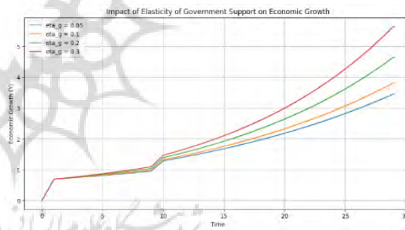
شکل ۵. شبیه‌سازی برای حالات مختلف \eta_g و شبیه‌سازی مونت کارلو با فاصله اعتماد ۹۵ درصد برای \eta_g با مقادیر پایه
