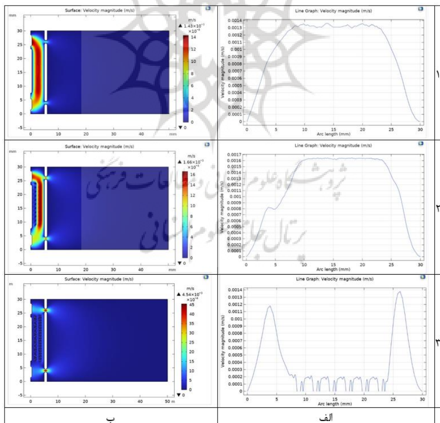
شکل ۶- الف) نمودار سرعت جریان سیال هوا درون پاکت ساختمانی دوپسته در سرعت ۱ متر بر ثانیه، ب) نحوه حرکت جریان سیال هوا درون پاکت ساختمانی دوپسته
