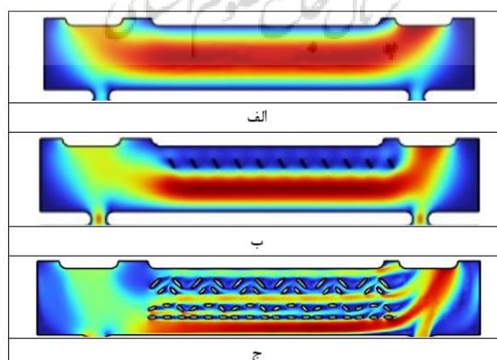
شکل ۱۸- نحوه عبور هوا در درون پاکت نمای دوپوسته با هندسه متفاوت، الف) هندسه ۱ ب) هندسه ۲ ج) هندسه ۳
