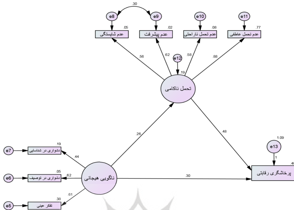
شکل ۱. مدل نهایی مسیرهای آزمون شده به همراه آماره‌های پیش‌بینی استاندارد شده پرخاشگری رقابتی در مسیر غیر مستقیم توسط متغیرهای نارسایی هیجانی و تحمیل ناکامی
