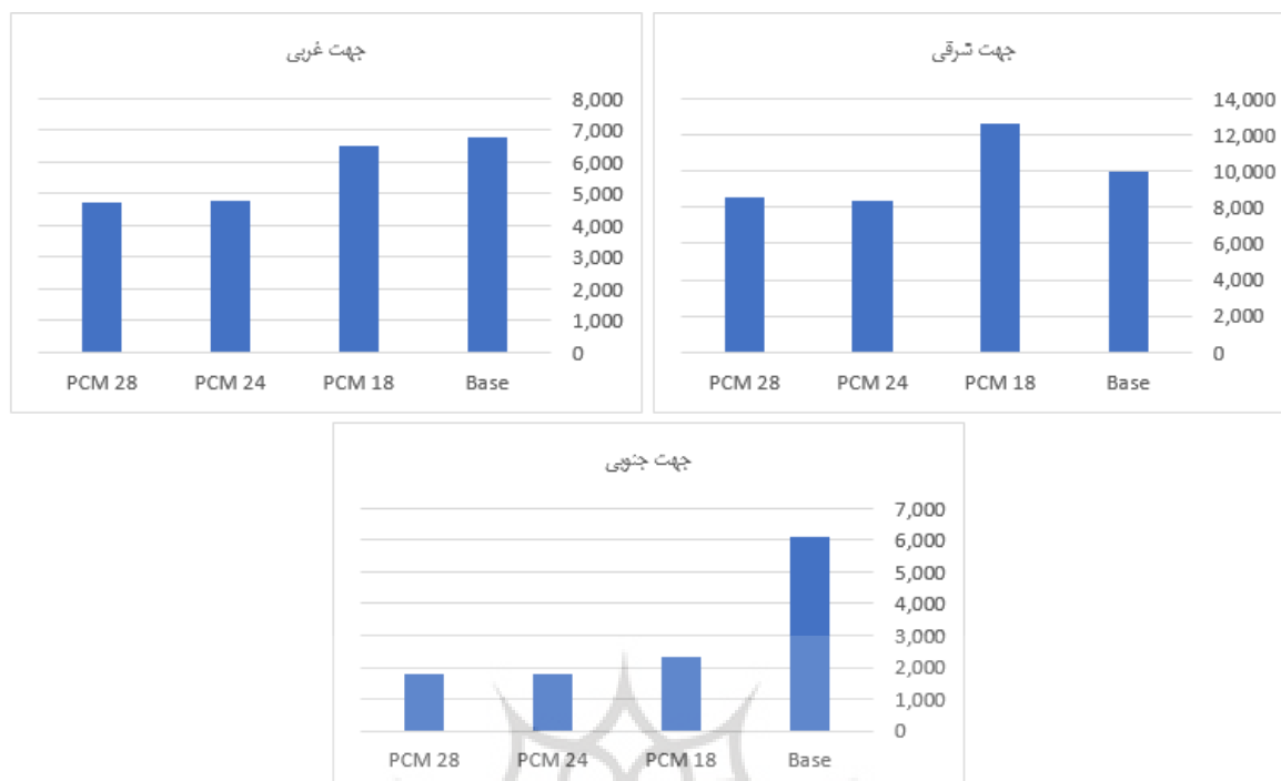
شکل ۸: مقایسه میزان مصرف انرژی در حالت پایه و دارای PCM در جهت‌های مورد بررسی در طی سال Fig 8: Comparison of the amount of energy consumption in the basic state and with PCM in the investigated directions during the year
