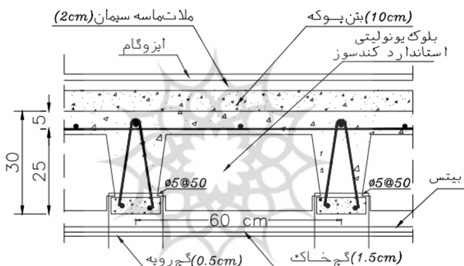
شکل ۲: جزئیات سقف طبقه پنجم Fig 2: Roof details of the fifth floor
