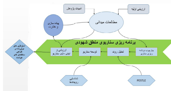
شکل ۳: مدل مفهومی
