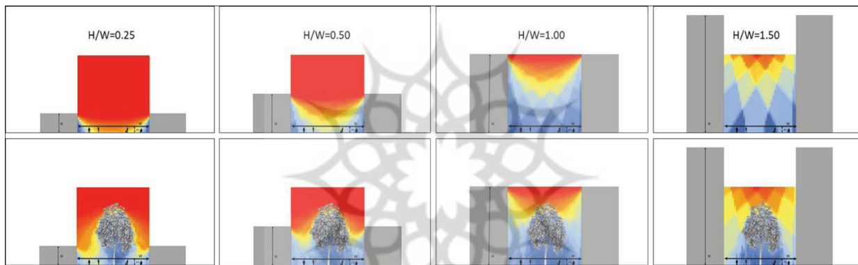
تصویر ۷- نمونه بصری فرضی تحلیل آسایش حرارتی با جهت‌گیری شمالی در اقلیم تهران در روز ۱ تیر (۲۲ ژوئن)
