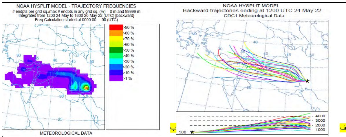
شکل ۵: الف) نقشه مسیر طوفان گرد و غبار، ب) تراکم طوفان گرد و غبار روز ۲۴ می ۲۰۲۲ در مسجدسلیمان
