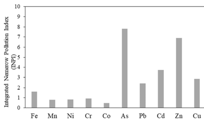
شکل ۴: نمودار میانگین فصلی شاخص جامع آلودگی نمره (INPI) برای فلزات سنگین در نمونه‌های گردوغبار منطقه مورد مطالعه. منبع: نگارندگان
