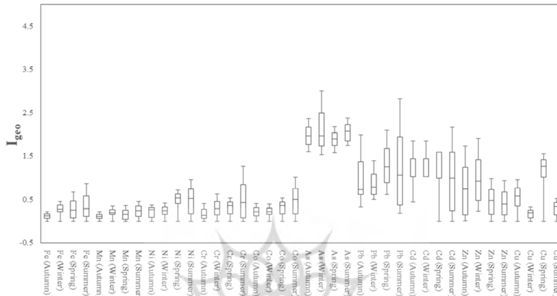
شکل ۹: نمودار جعبه‌ای شاخص زمین‌انباشتگی ( I_{geo} ) عناصر سنگین در نمونه‌های گردوغبار منطقه مورد مطالعه به تفکیک چهار فصل.
