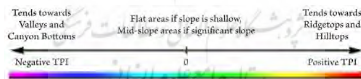
شکل ۲. مقادیر شاخص موقعیت توپوگرافیک و نوع لندفرم
