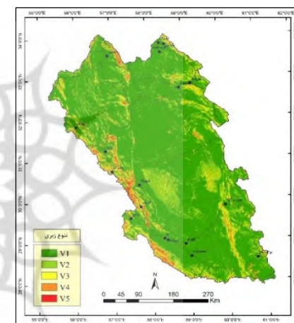
شکل ۹. تنوع زبری ناهمواری (Rgv) حوضه لوت
