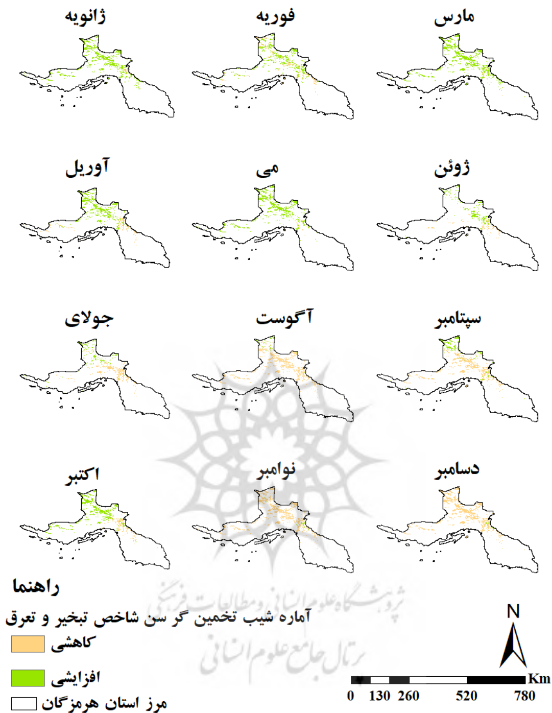
شکل ۱۰. روند تغییرات شاخص تبخیر و تعرق واقعی بر اساس شیب تخمین گر سن در بازه زمانی ۲۰۰۱-۲۰۲۲ منبع: (یافته‌های پژوهش)
