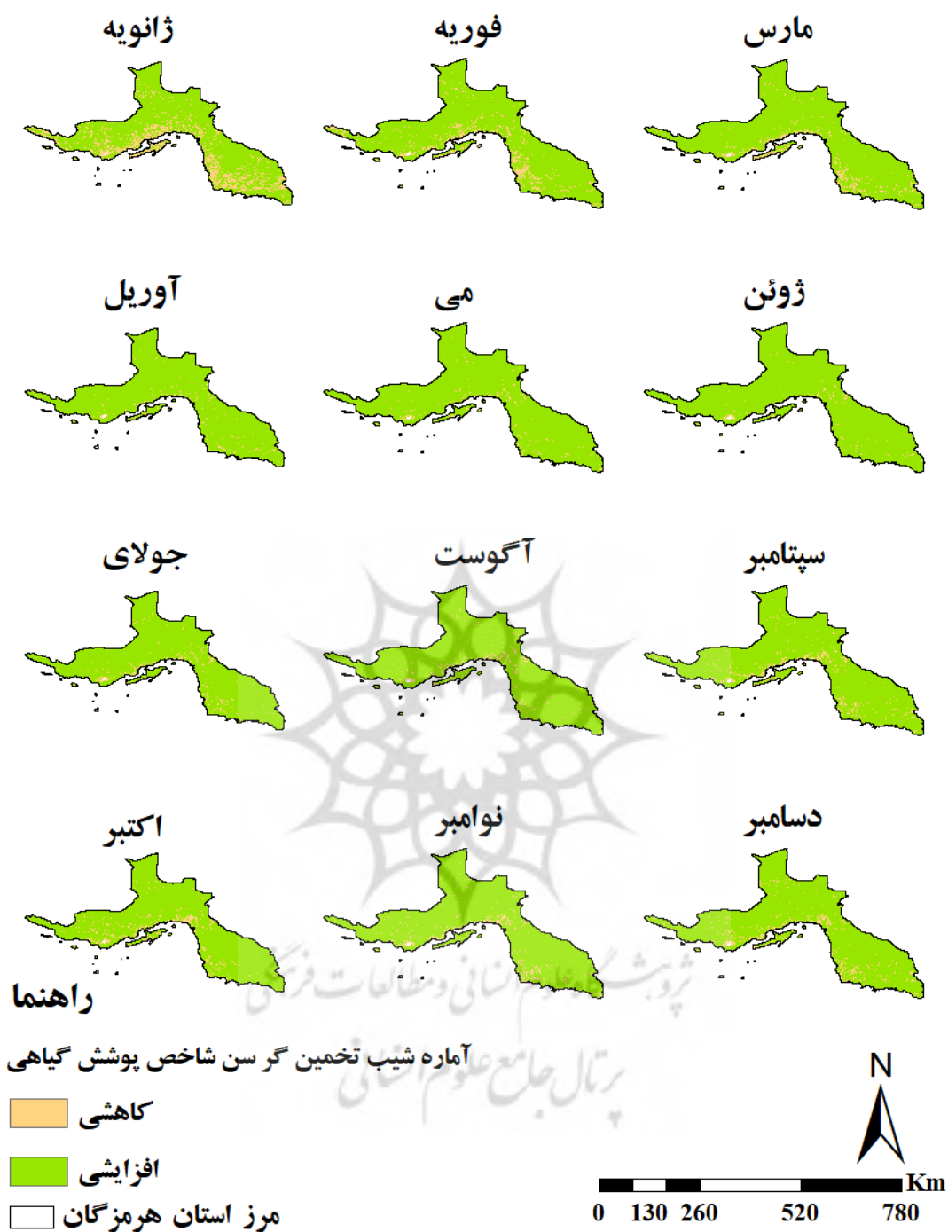
شکل ۸. روند شاخص پوشش گیاهی NDVI بر اساس شیب تخمین گرسن در بازه زمانی ۲۰۰۱-۲۰۲۲
