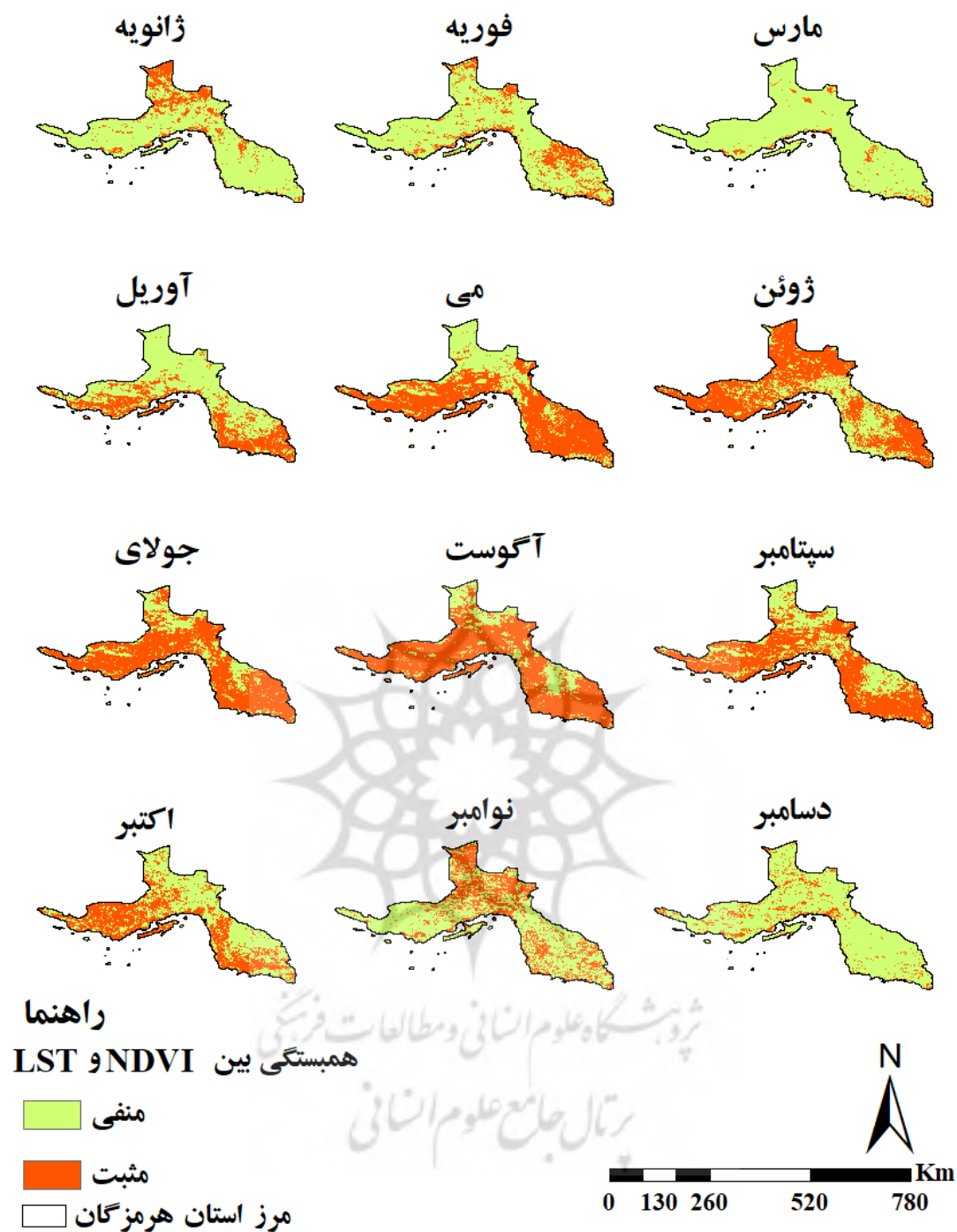
شکل ۱۶. همبستگی بین شاخص پوشش گیاهی NDVI و LST در بازه زمانی ۲۰۲۲-۲۰۰۱
