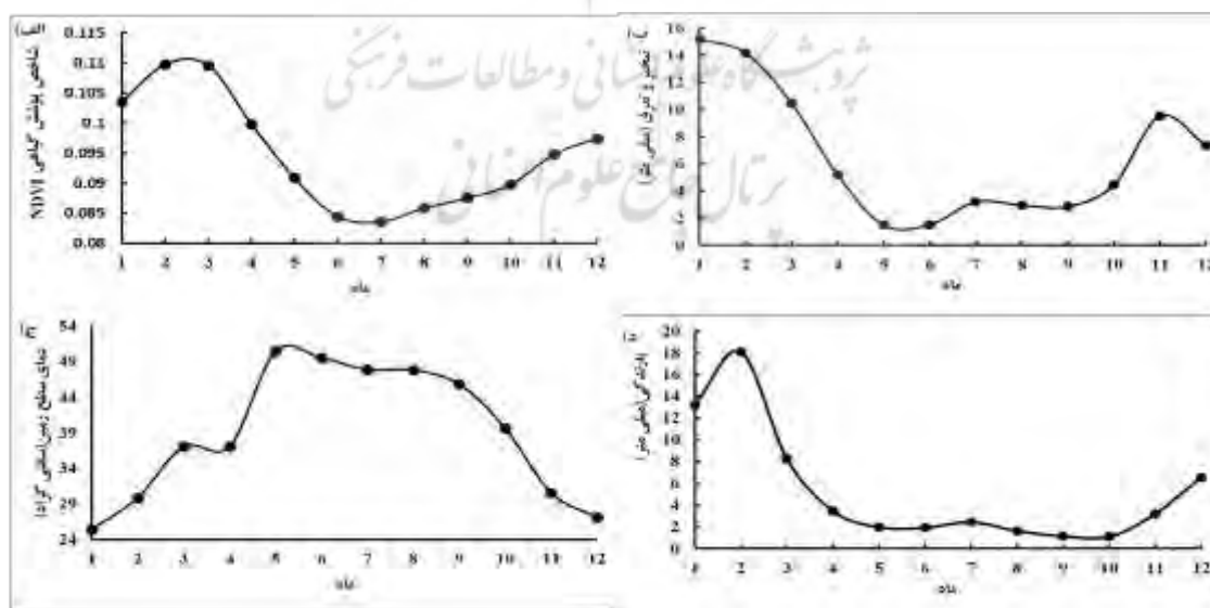
شکل ۲. تغییرات متوسط شاخص‌های NDVI، ET، LST و بارندگی به ترتیب الف، ب، ج و د در بازه زمانی ۲۰۰۱-۲۰۲۲ استان هرمزگان منبع: (یافته‌های پژوهش)
