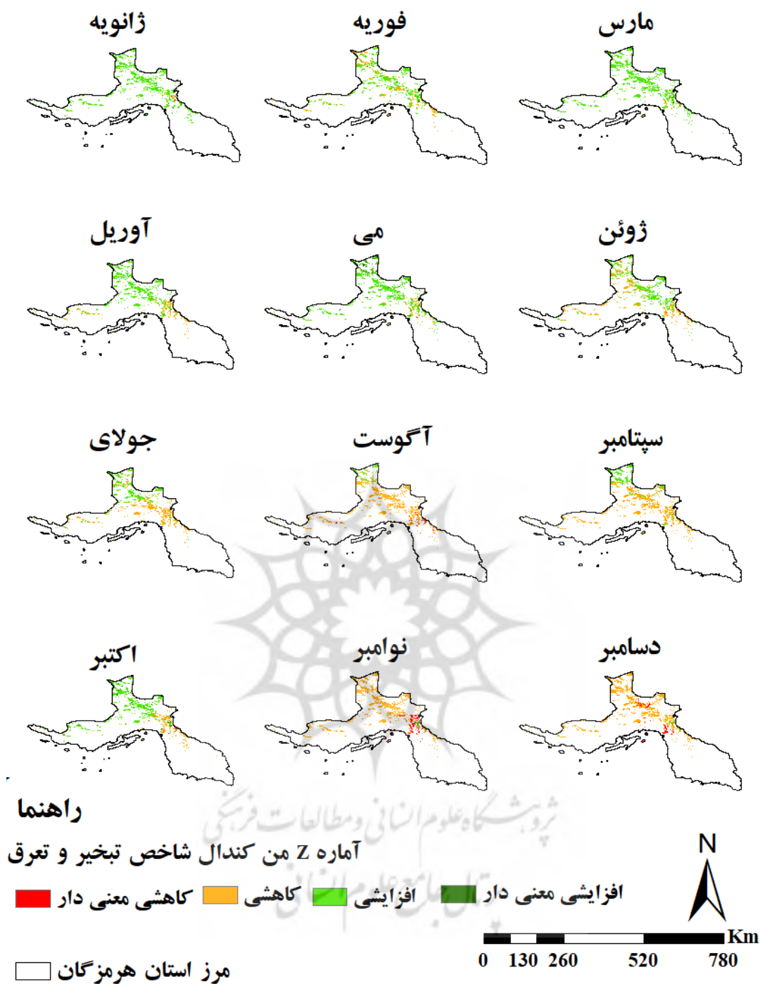
شکل ۹. روند تغییرات شاخص تبخیر و تعرق واقعی بر اساس آزمون‌های من-کندهال در بازه زمانی ۲۰۰۱-۲۰۲۲ منبع: (یافته‌های پژوهش)
