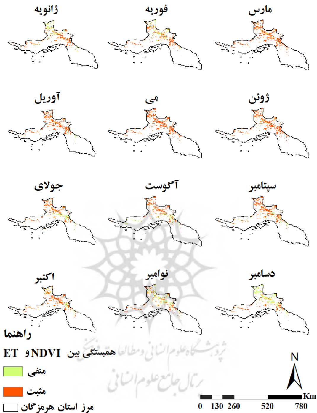
شکل ۱۵. همبستگی بین شاخص پوشش گیاهی ET و NDVI در بازه زمانی ۲۰۰۱-۲۰۲۲
