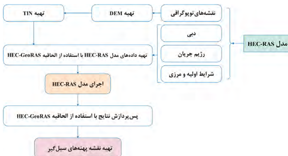
شکل ۲. فلوچارت مدل‌سازی سیلاب با استفاده از مدل HEC-RAS
