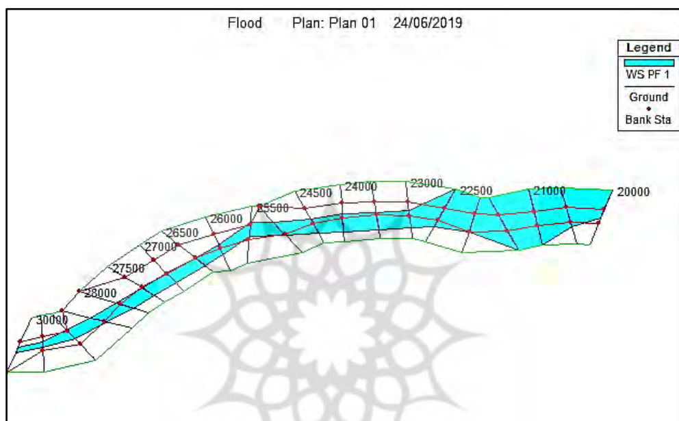
شکل ۴. شبیه‌سازی سیلاب با دوره بازگشت ۲۵ سال برای قسمتی از بازه دوم در نرم‌افزار HEC-RAS
