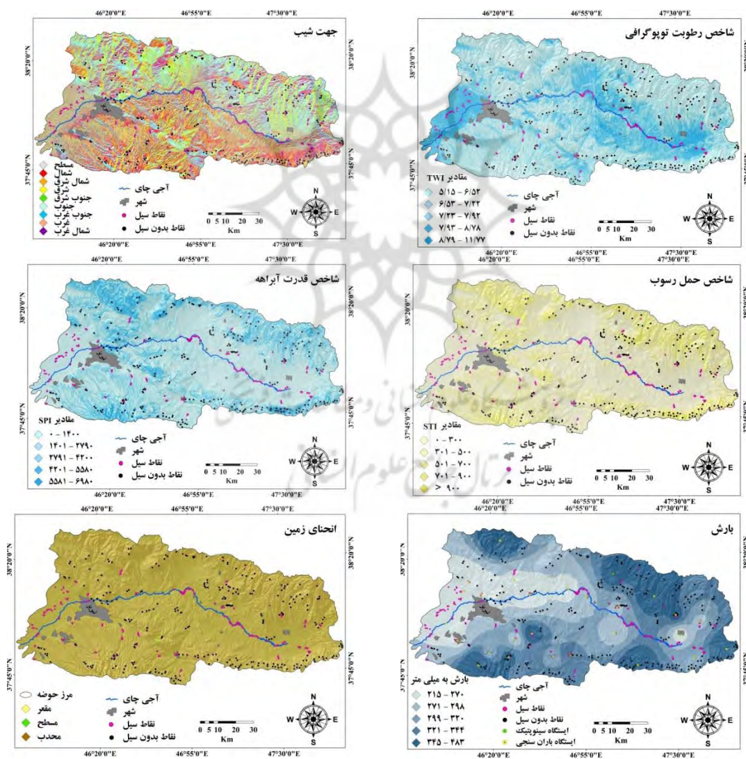
شکل ۳: نقشه پارامترهای مورد استفاده در تحقیق
