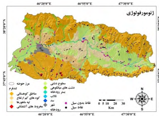
ادامه شکل ۳: نقشه پارامترهای مورد استفاده در تحقیق
