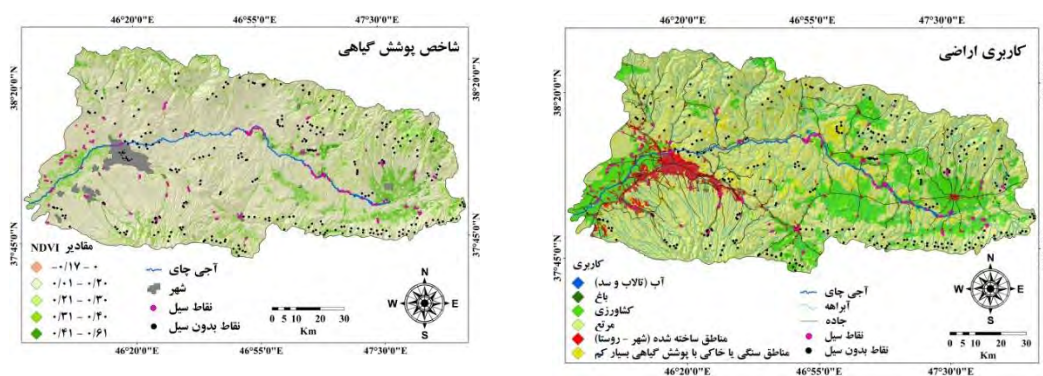
ادامه شکل ۳: نقشه پارامترهای مورد استفاده در تحقیق
