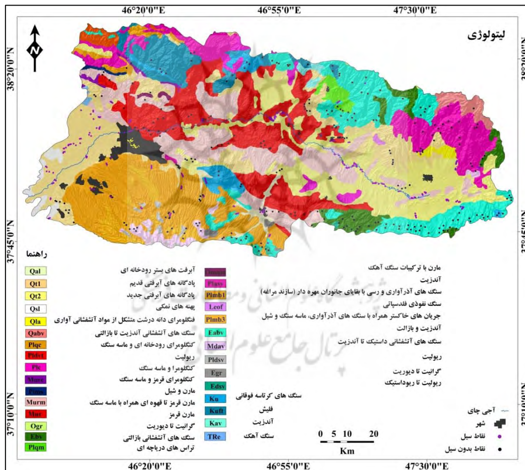
شکل ۴: نقشه لیتولوژی حوضه آبریز آجی جای
