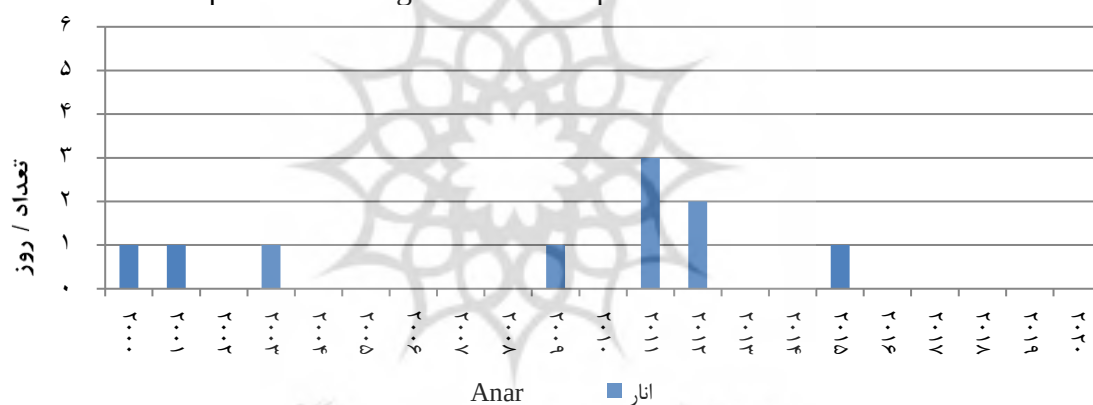
شکل ۴- مجموع سالانه فراوانی رخداد گردوغبار برای ایستگاه انار طی دوره آماری ۱۳۷۹-۱۳۹۹
