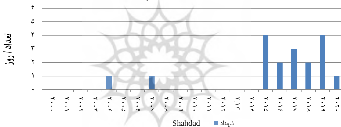
شکل ۱۲- مجموع سالانه فراوانی رخداد گردوغبار برای ایستگاه شهداد طی دوره آماری ۱۳۷۹ - ۱۳۹۹
