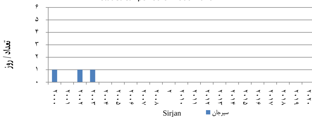
شکل ۱۱- مجموع سالانه فراوانی رخداد گردوغبار برای ایستگاه سیرجان طی دوره آماری ۱۳۷۹ - ۱۳۹۹
