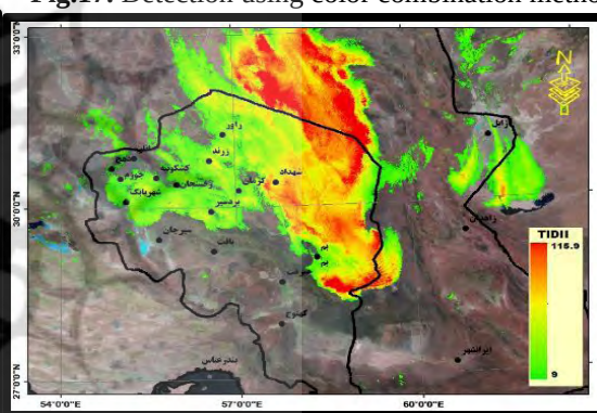
شکل ۱۹- آشکارسازی با استفاده از الگوریتم TIIDI
