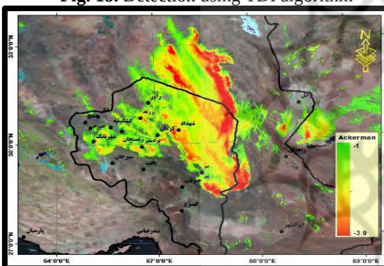
شکل ۲۰- آشکارسازی با استفاده از الگوریتم Ackerman
