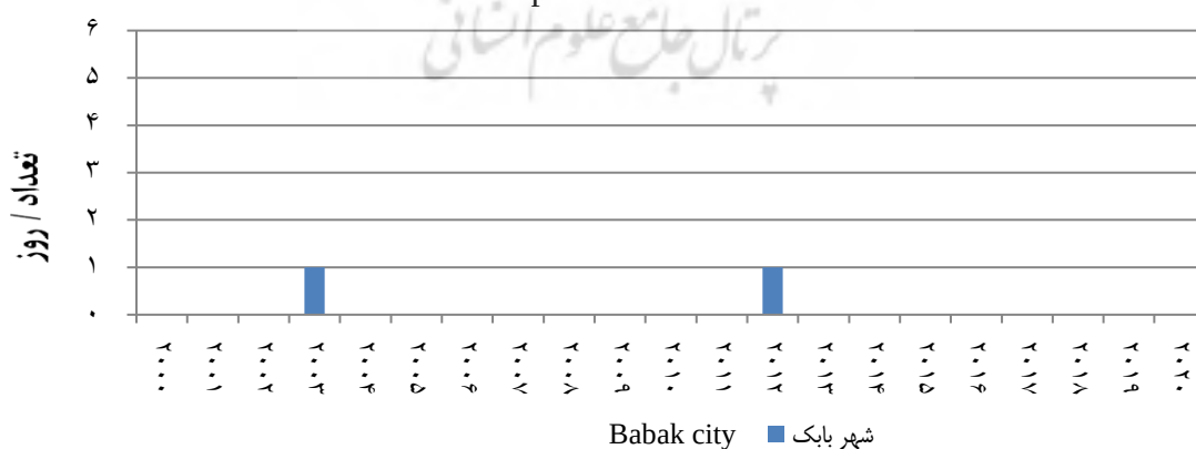
شکل ۱۳- مجموع سالانه فراوانی رخداد گردوغبار برای ایستگاه شهر بابک طی دوره آماری ۱۳۷۹ - ۱۳۹۹
