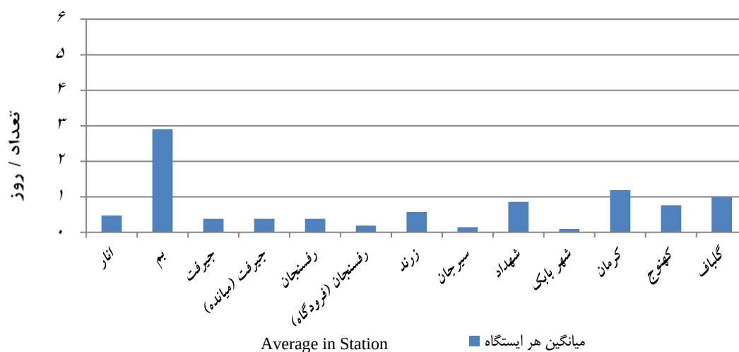
شکل ۳- میانگین سالانه فراوانی رخداد گردوغبار برای ایستگاه‌های استان کرمان طی دوره آماری ۱۳۷۹-۱۳۹۹
