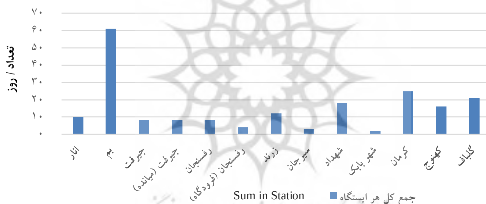
شکل ۲- مجموع سالانه فراوانی رخداد گردوغبار برای ایستگاه‌های استان کرمان طی دوره آماری ۱۳۷۹-۱۳۹۹
