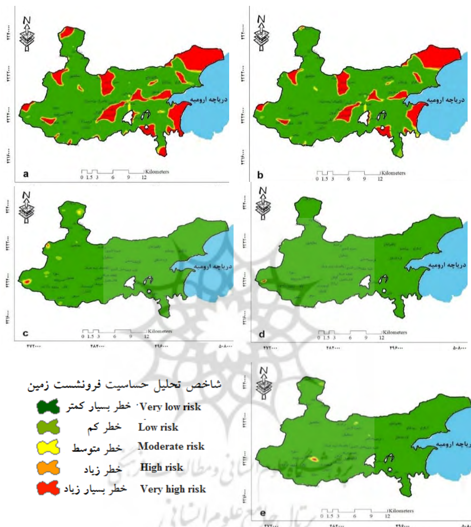
شکل ۳- نقشه تحلیل حساسیت فرونشست، با استفاده از مدل ANFIS در پنج تابع عضویت به ترتیب: a تابع عضویت دوزنقه‌ای، b تابع عضویت مثلثی، c تابع عضویت گوسی، d تابع عضویت گوسی دوطرفه، e تابع عضویت منحنی زنگوله
