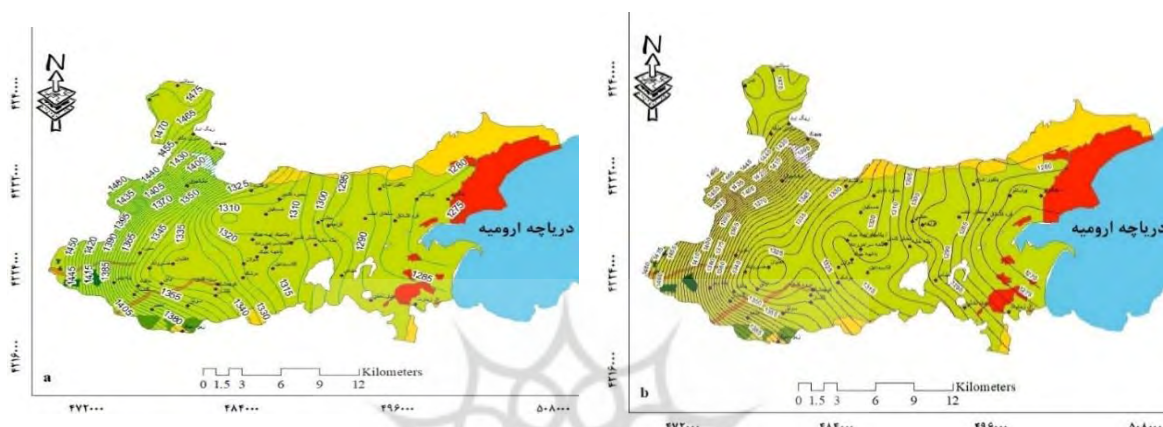
شکل ۶- نقشه ایزوپیز حداکثر (a) و ایزوپیز حداقل (b)
