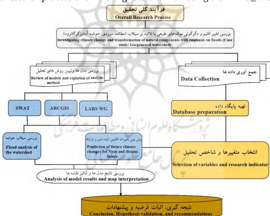
شکل ۳- فرایند تحقیق پهنه بندی منطقه ای سیلاب با استفاده از مدل هیدرولوژیکی SWAT
