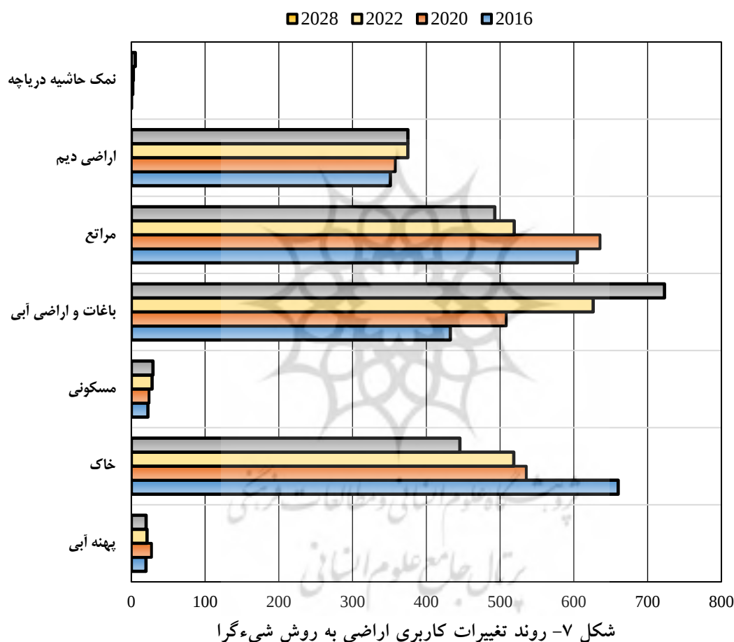
شکل ۷- روند تغییرات کاربری اراضی به روش شیء‌گرا
