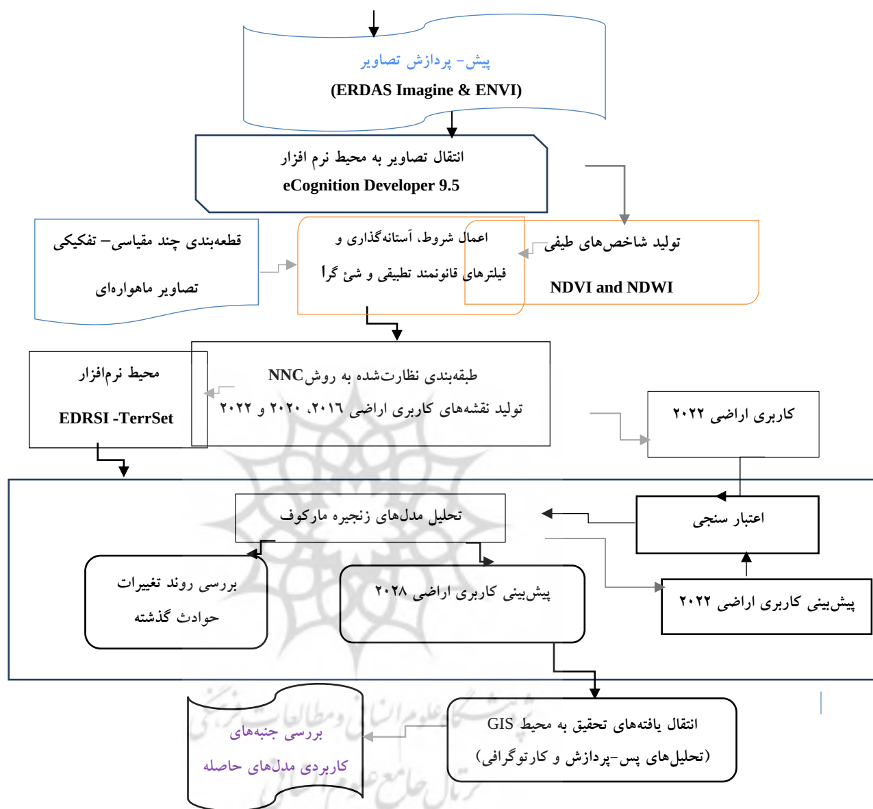
شکل ۲- نمودار جریانی مراحل انجام تحقیق
