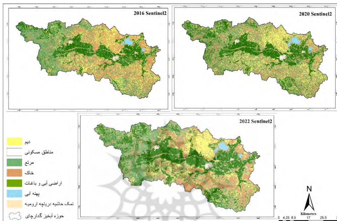
شکل ۴- نقشه کاربری اراضی برای سال‌های موردبررسی در حوزه آبخیز گدارچای-دریاچه ارومیه
