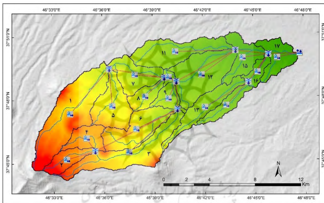
شکل ۷- شماتیک حوضه اوجان‌چای در محیط اکستنشن EEC-GooMMS همراه با نام زیرحوضه‌ها
