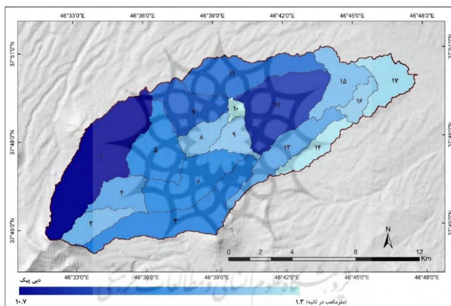
شکل ۱۱- دبی پیک زیرحوضه‌های اوجان‌چای برای بارش با دوره بازگشت ۱۰ ساله (حدود ۳۴ میلی‌متر)
