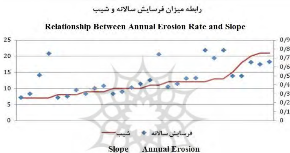
شکل ۶- رابطه بین شیب محل برداشت نمونه ریشه و نرخ فرسایش سالانه
