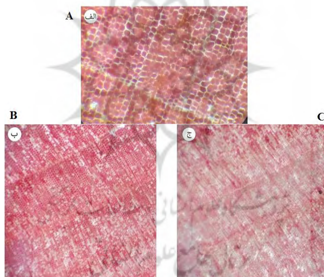
شکل ۴- مطالعه حلقه های رویشی با میکروسکوپ نوری با بزرگنمایی ۳۰. در تصویر الف که قبل از برون زدگی ریشه است سلول های آوندی نظم معینی داشته در تصویر ب و ج که بعد از برون زدگی گرفته شده است نظم، تراکم و اندازه سلول ها از بین رفته است.
