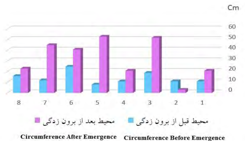
شکل ۸- مقایسه میانگین محیط و مساحت آوندها در حلقه‌های رشد قبل و بعد از بیرون زدگی از خاک
