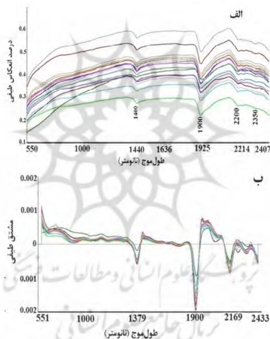
شکل ۸. طیف بازتابی خام (الف) و مشتق اول (ب) از هفده نمونه خاک
