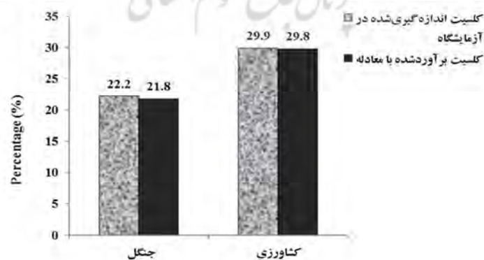
شکل ۷. مقایسه میانگین کلسیت اندازه‌گیری شده در آزمایشگاه و برآورد شده با معادله حاصل از تصویر ماهواره‌ای در دو کاربری
