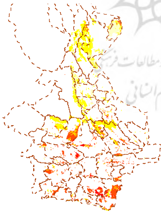
شکل ۸. میزان همبستگی میان VHI و TSDI
