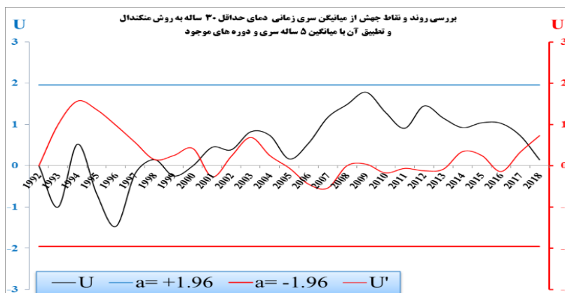
شکل (۹). روند تغییرات حداقل دما در ایستگاه ژونفیزیک
