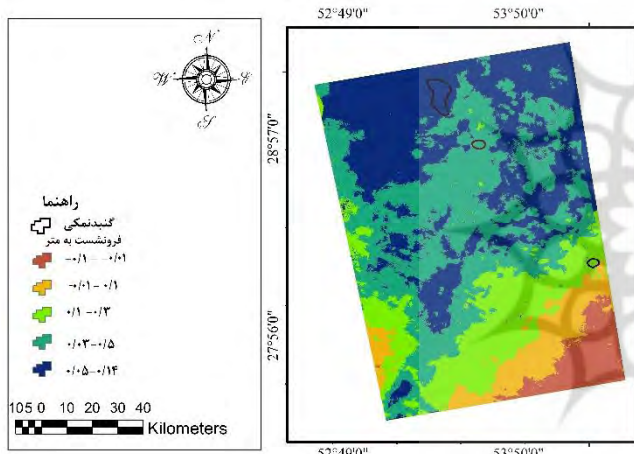
شکل (۴). فرونشست گنبد های نمکی شهرستان فسا
