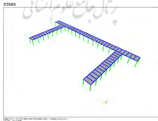
شکل ۵. هندسه سه بعدی مدل
