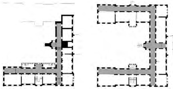
شکل ۳. جانمایی راهروهای ساختمان دانشکده معماری و شهرسازی، راست: پلان طبقه همکف-چپ: پلان طبقه زیرزمین منبع: برگرفته از نارنجی، ۱۳۹۸
