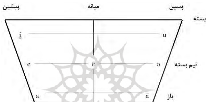
شکل ۲- نمودار واکه‌های گویش عبدالملکی
