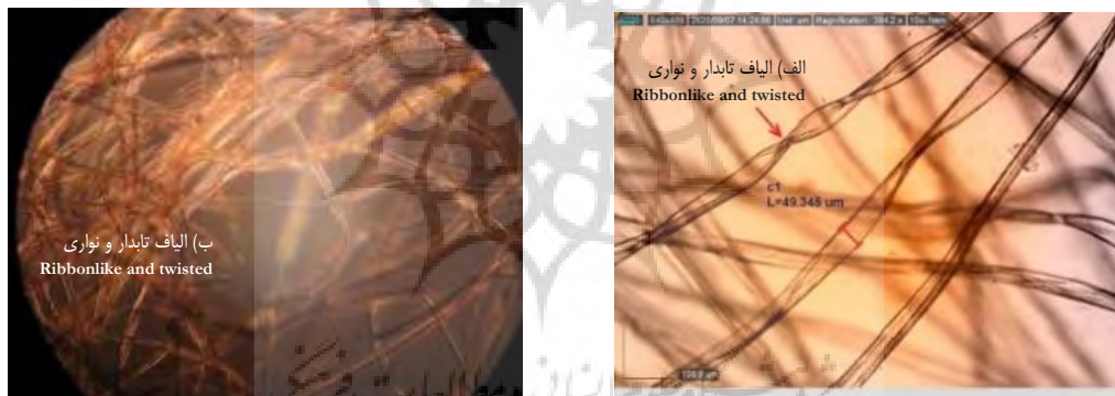
شکل ۱۰: الیاف لینت پنبه در بزرگنمایی ۲۰۰X: الف) میکروسکوپ نوری و ب) با میکروسکوپ پلاریزان Fig. 10: Cotton lint fibers at x200 magnification: a) with light and b) polarized microscopic
