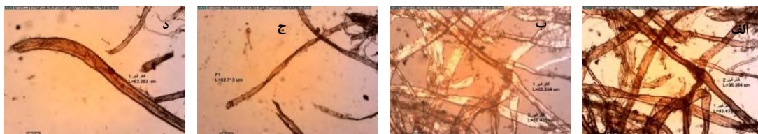
شکل ۱۳: الیاف پوستی کتان و پنبه در خمیر کاغذ دولت‌آبادی ۳۶۰۵ (قرن ۷ ق.ه.ق): الف) الیاف پنبه و کتان با آماس، ب) الیاف در نور پلاریزان، ج) الیاف روبان مانند پنبه (لینت)، د) الیاف ضخیم و استوانه‌ای پنبه (لینتر)
