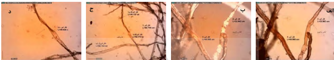
شکل ۱۴: الیاف پوستی کتان و لنت پنبه در خمیر کاغذ دولت‌آبادی (قرن ۸ ه. ق): الف) ضخامت‌های مختلف و حفره لومن باریک و حضور آماس، ب) بندها در نور پلاریزان، ج) الیاف پنبه و کتان و د) الیاف پنبه
