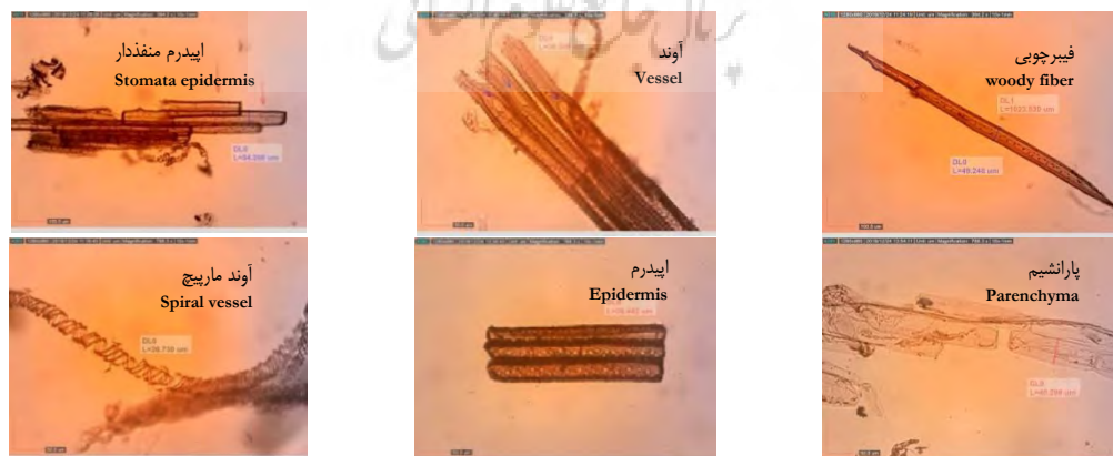
شکل ۱: الیاف چوبی و سلول‌های همراه کتان با میکروسکوپ نوری با بزرگنمایی 100\times و 200\times Fig. 1: Woody fibers and associated cells of flax with light microscopic at 100\times and 200\times magnification
