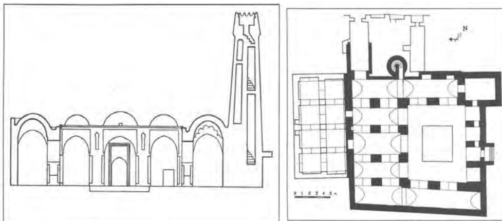
شکل ۱- پلان و برش بنا
