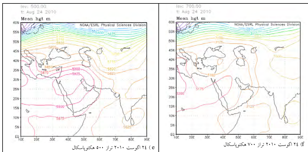
شکل ۴. نقشه هم ارتفاع ژئوپتانسیل تراز ۵۰۰ و ۷۰۰ هکتوپاسکال در روزهای ۲۲، ۲۳ و ۲۴ اگوست ۲۰۱۰
