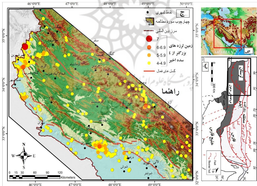
شکل ۱. موقعیت جغرافیایی، زمین‌ساختی و لرزه زمین‌ساختی منطقه مورد مطالعه (الف): سایت مؤسسه ژئوفیزیک دانشگاه تهران ۱ ؛ ب: برگرفته از (Masoudi et al, ۲۰۱۵: ۳۰۳۲)؛ ج: ترسیم: نگارندگان
