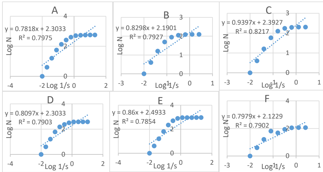
شکل ۷. نمودار \text{Log-Log} معکوس طول ضلع شبکه و تعداد خانه‌های حاوی رومرکز زمین لرزه (۱۹۰۰ تا ۲۰۲۰) بدون بزرگای
