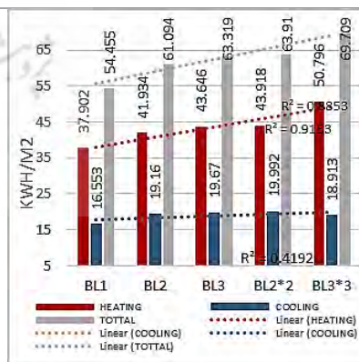
تصویر ۹- میزان مصرف انرژی گرمایشی، سرمایشی و نهایی سالانه تمام گویها
