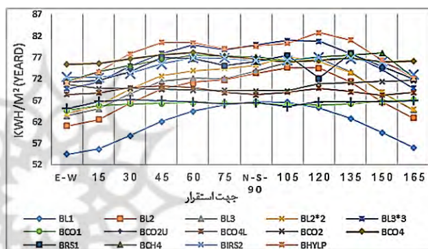
تصویر ۸- نمودار میزان مصرف انرژی در جهات مختلف استقرار گویهای پانزده‌گانه
