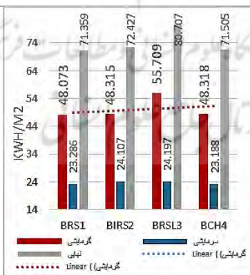
تصویر ۹- میزان مصرف انرژی گرمایشی، سرمایشی و نهایی سالانه تمام گویها
