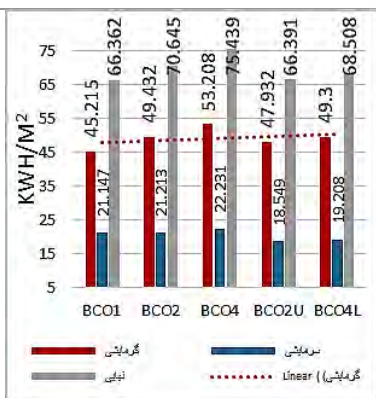
تصویر ۹- میزان مصرف انرژی گرمایشی، سرمایشی و نهایی سالانه تمام گویها
