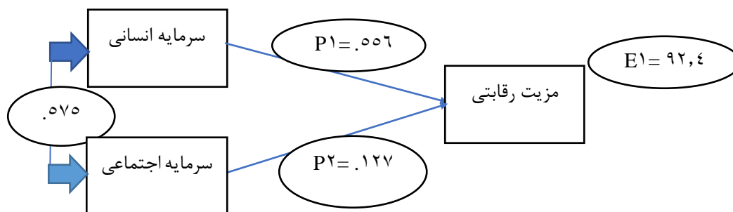
نمودار (۱) تجزیه و تحلیل مسیر
