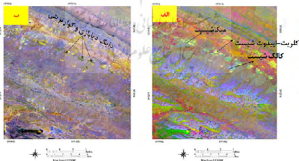
شکل ۸. نتایج تحلیل مولفه اصلی بر روی ۹ باند سنتینل ۲. ترکیب رنگین PC4, PC5, PC8 و تفکیک میکاشیست، کلریت-اپیدوت شیست و کالک شیست (الف) و آشکارسازی واحدهای دایک دیابازی با ترکیب رنگی PC4, PC2, PC3 (ب).
