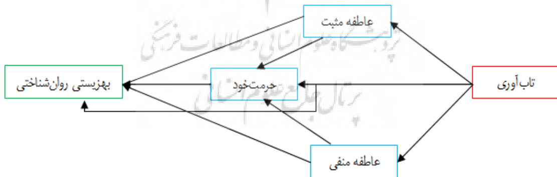
شکل ۱. نمودار علی
